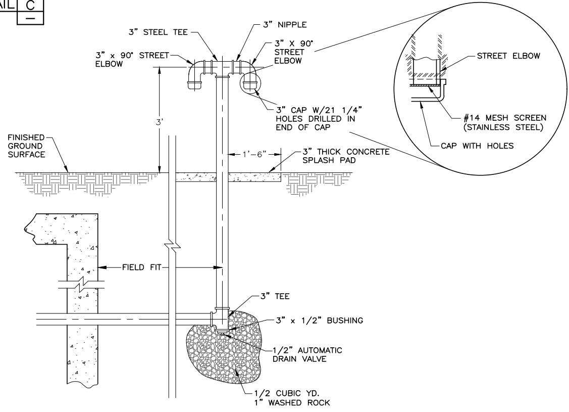
PRESSURE RELIEF PIPE N.T.S.
